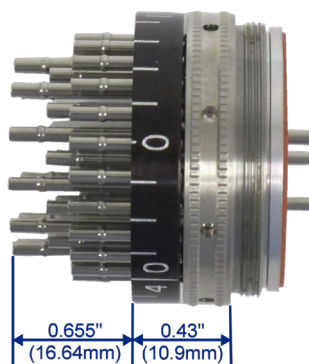
48DM-1/2 (Male)
